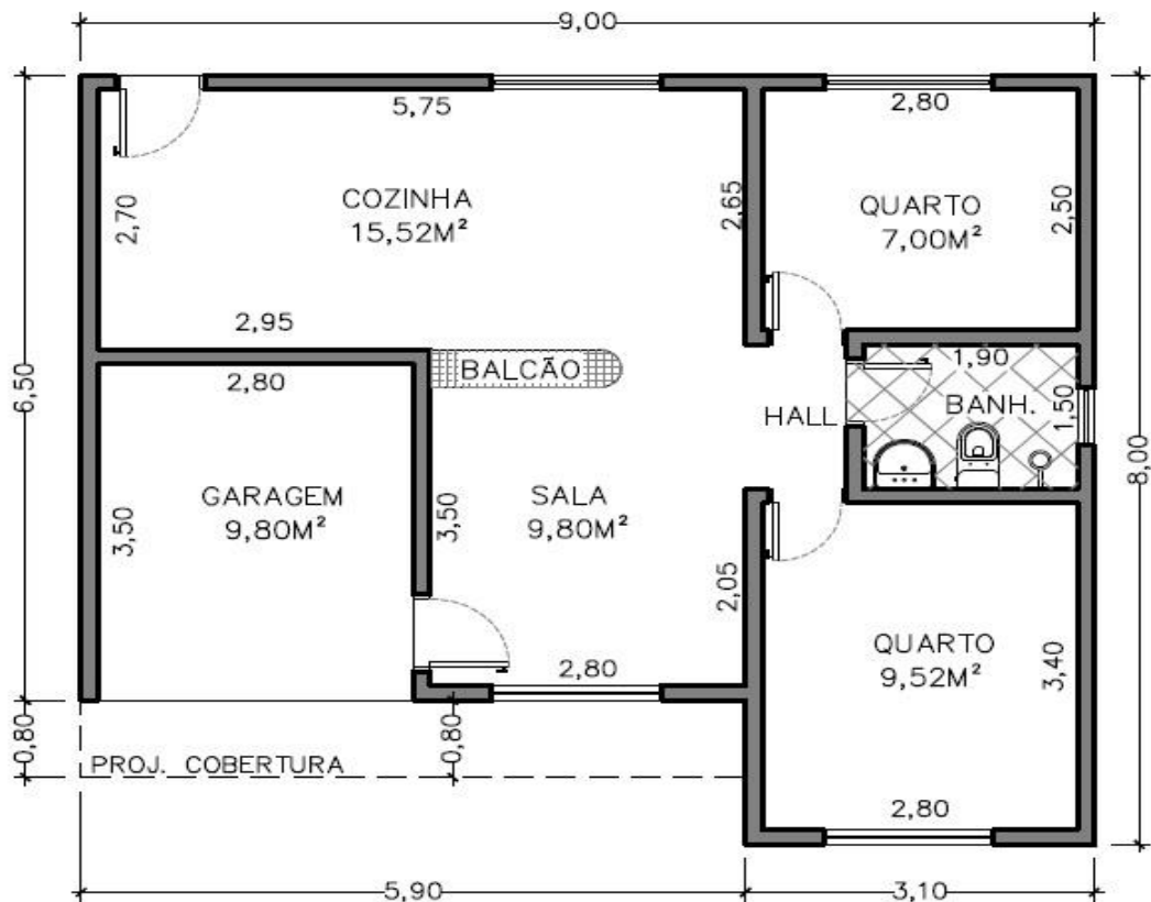
01 PLANTA BAIXA – 67,87M 2 ESCALA 1: 75
